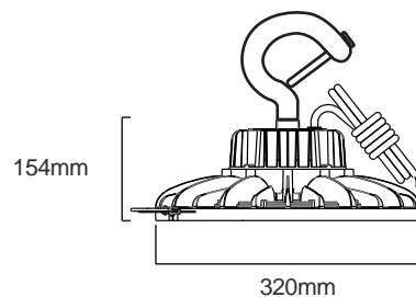
240W: \phi 320 \times 154 mm
